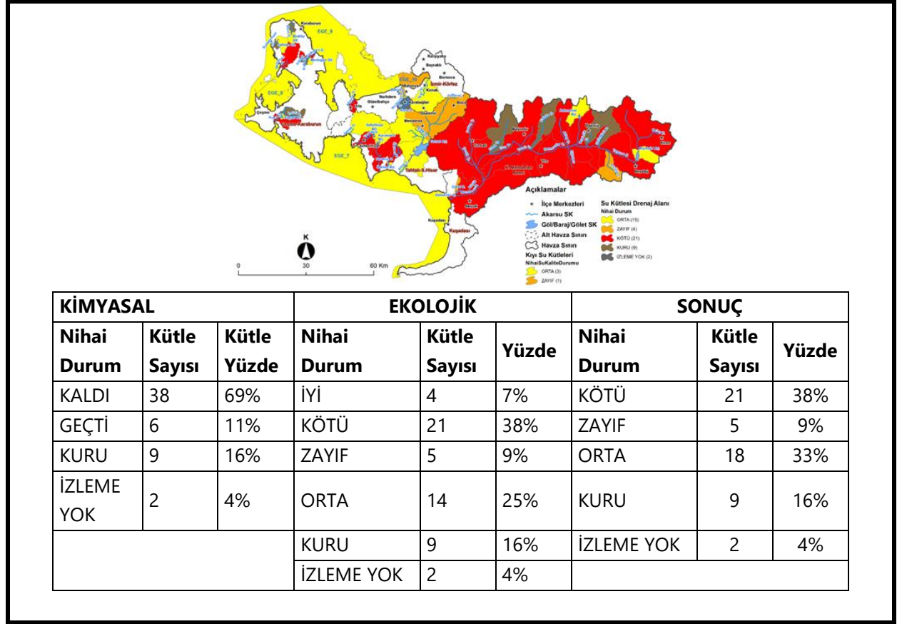
Şekil 8. Küçük Menderes Havzası YÜS kütleleri nihai durumu (SYGM, 2018b)
