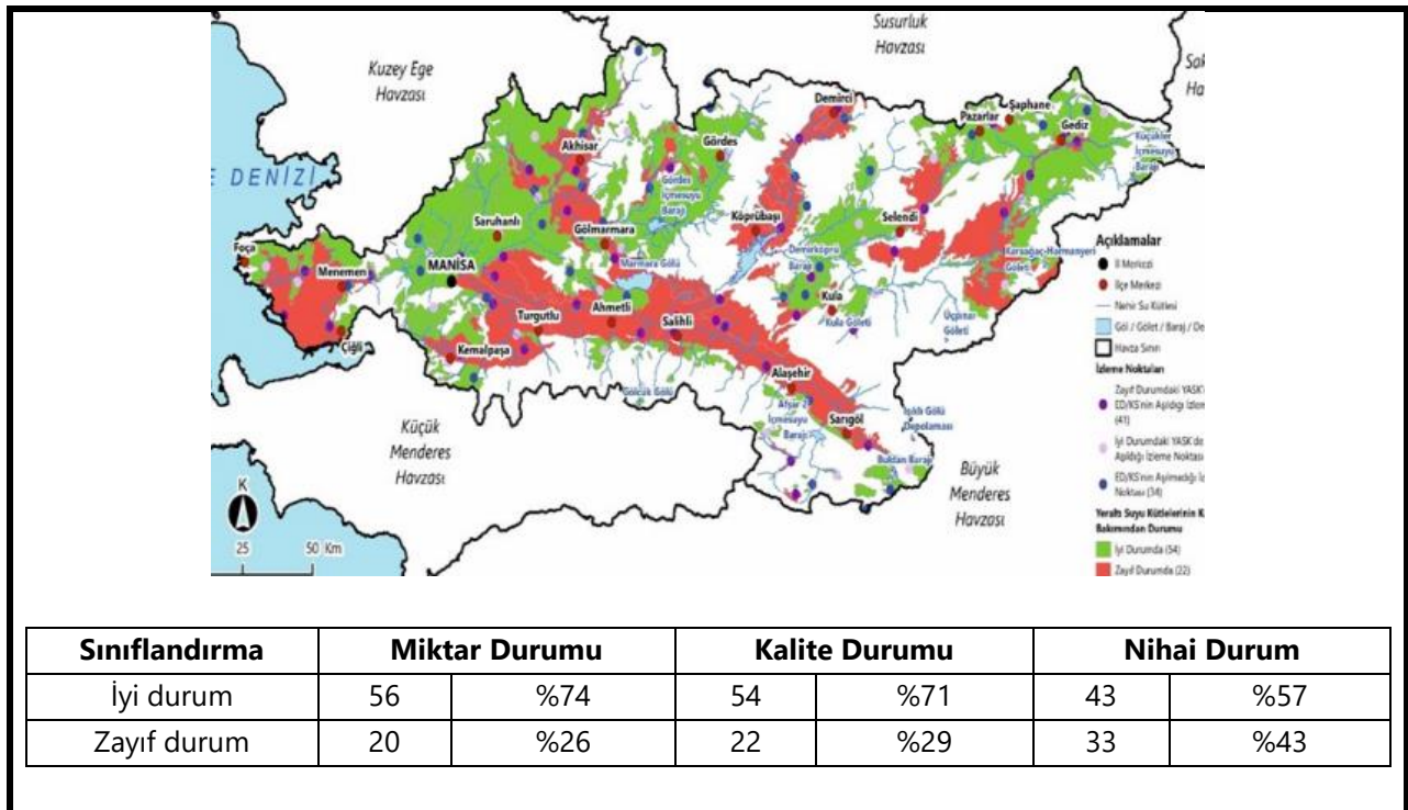
Şekil 6. Gediz Havzası YAS kütelleri miktar ve kalite durumu (SYGM, 2018a; SYGM, 2023)
