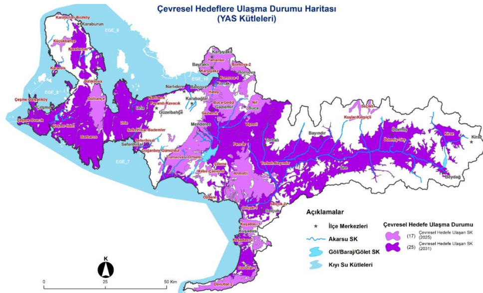
Şekil 10. Küçük Menderes Havzası YAS kütleleri çevresel hedeflere ulaşma haritası ((SYGM, 2018a)
