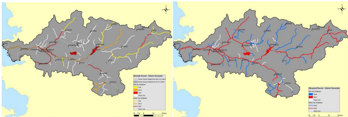
Şekil 4. Gediz Havzası YÜS kütleleri izleme sonuçları (sol: ekolojik, sağ: kimyasal) (SYGM, 2023)
